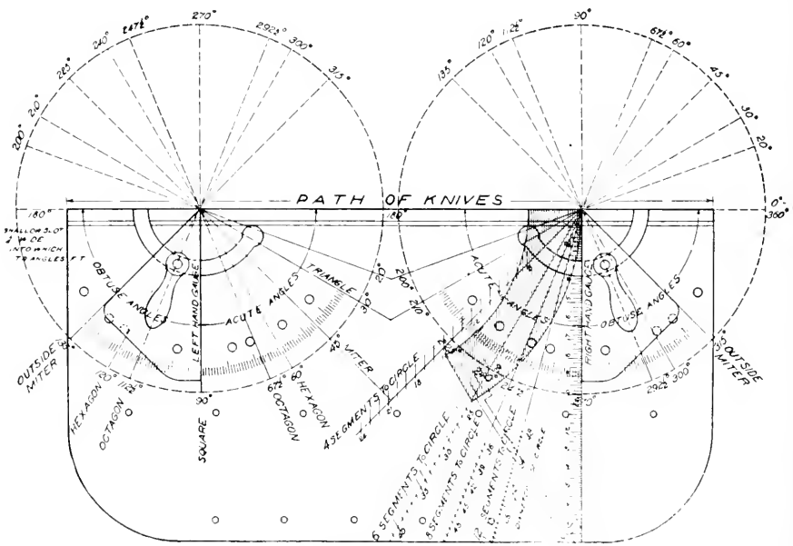
FIG. 209. TRIMMER TABLE.
